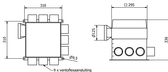
Homebox Delta EC – avec 9 connections Ventoflex
