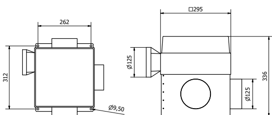
Homebox Delta EC – avec brides
