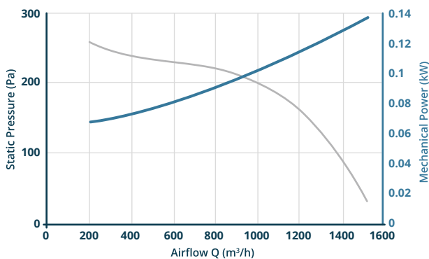
DAC/W2200/4 S
